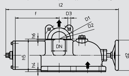
Konstrukcja zaworu - Powrót do zbiornika - bez pokrętła
