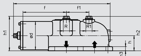
Konstrukcja zaworu - Cyrkulacyjna - bez pokrętła
